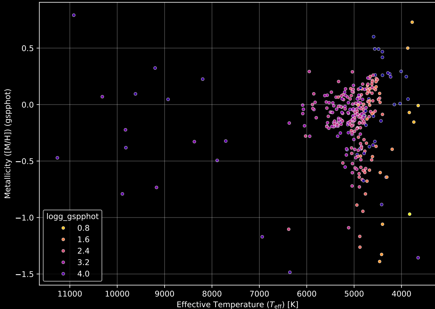
APOGEE DR17 Field: [160-12] Stellar Population Parameters (n= 311)
